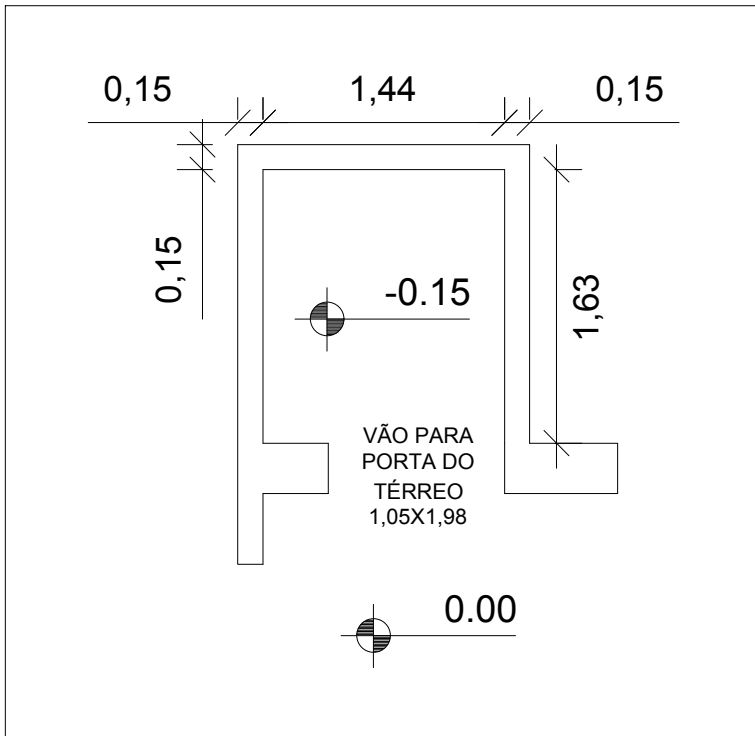
PLANTA BAIXA DO TÉRREO
