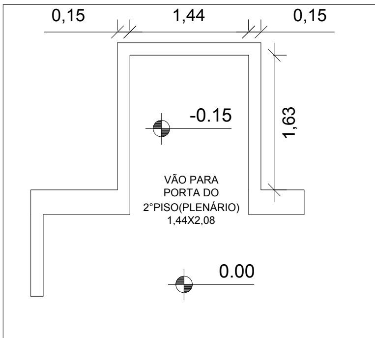
PLANTA BAIXA DO 2º PISO
